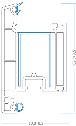
60 - ODS - C 60 - Outward Door Sash
