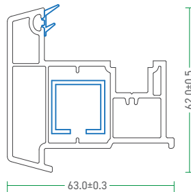
60 - FM - B 60 - Fly Mullion Euro Groove
