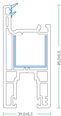
92 - SDS - C 92 - Sliding Sash - Door
