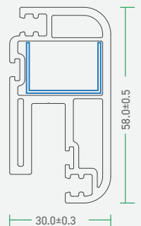
92 - MDS - C 92 - Mesh Door Sash
