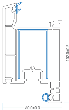
60 - IDS - C 60 - Inward Door Sash
