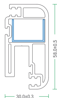
92 - MDS - C 92 - Mesh Door Sash
