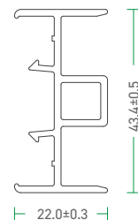
92 - IAD - A 92 - Inline Adapter Door
