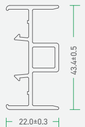
92 - IAD - A 92 - Inline Adapter Door
