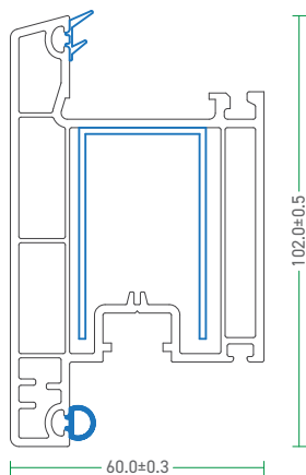
60 - ODS - B 60 - Outward Door Sash
